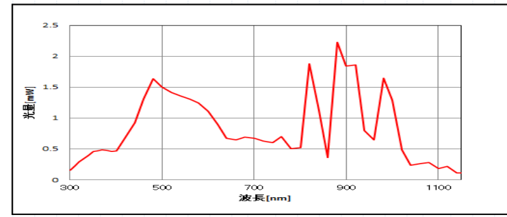
* 波長純度20nm選択時 バンドルファイバφ3mm 全光束入射時において *
