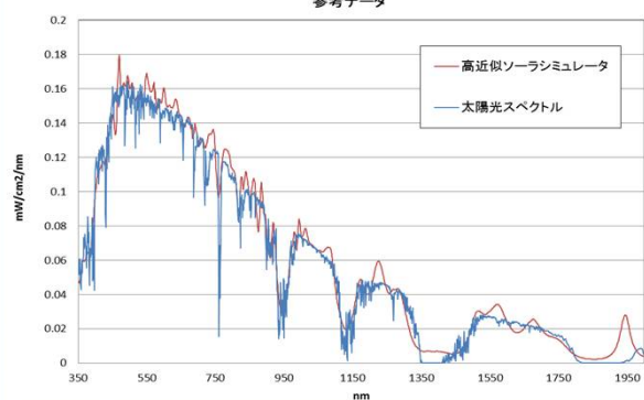
ソーラシミュレータのスペクトル
